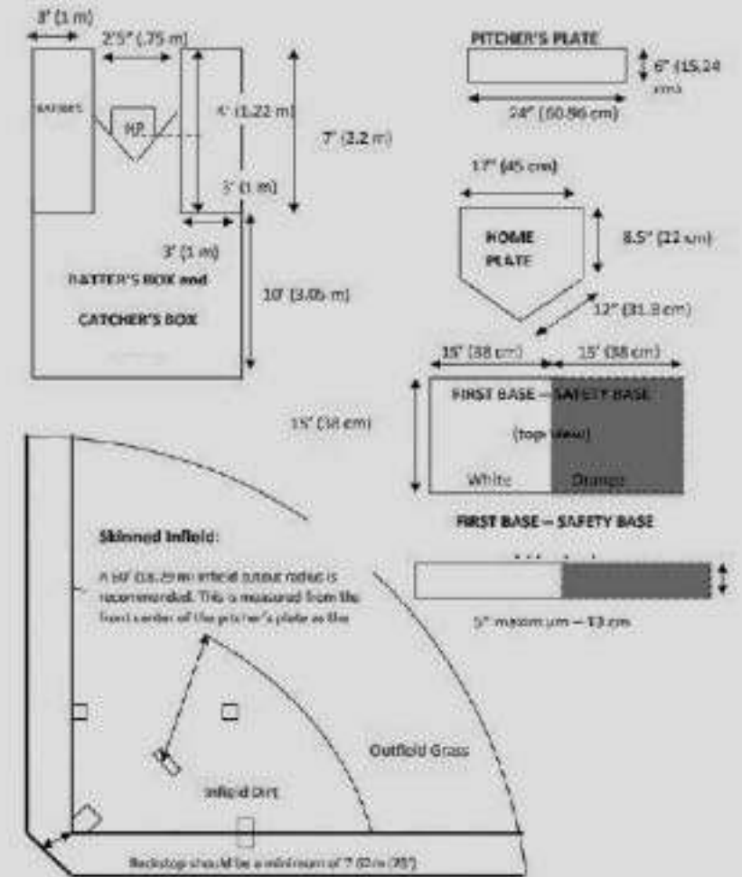
Figura 47. Dimensiones. Fuente: Guía de diseño de instalaciones deportivas.
