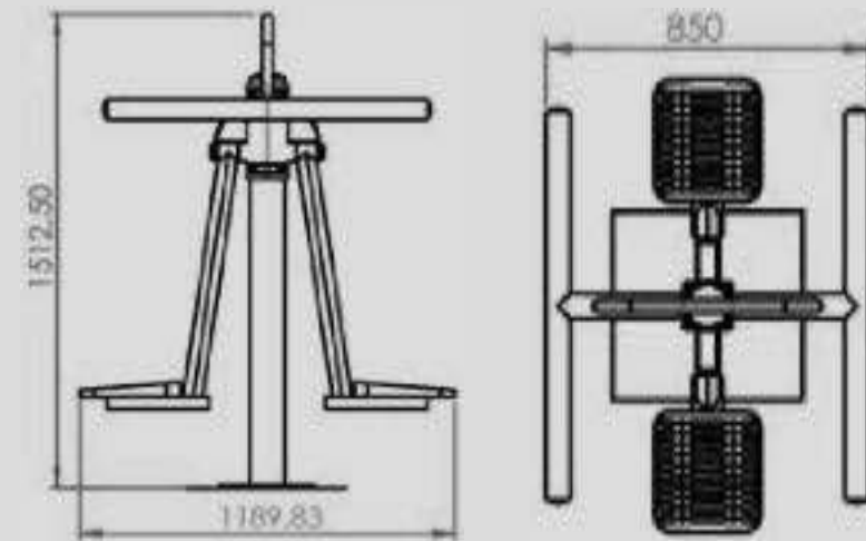
Figura 34. Dimensiones El Surf. Fuente: Equidesa.
