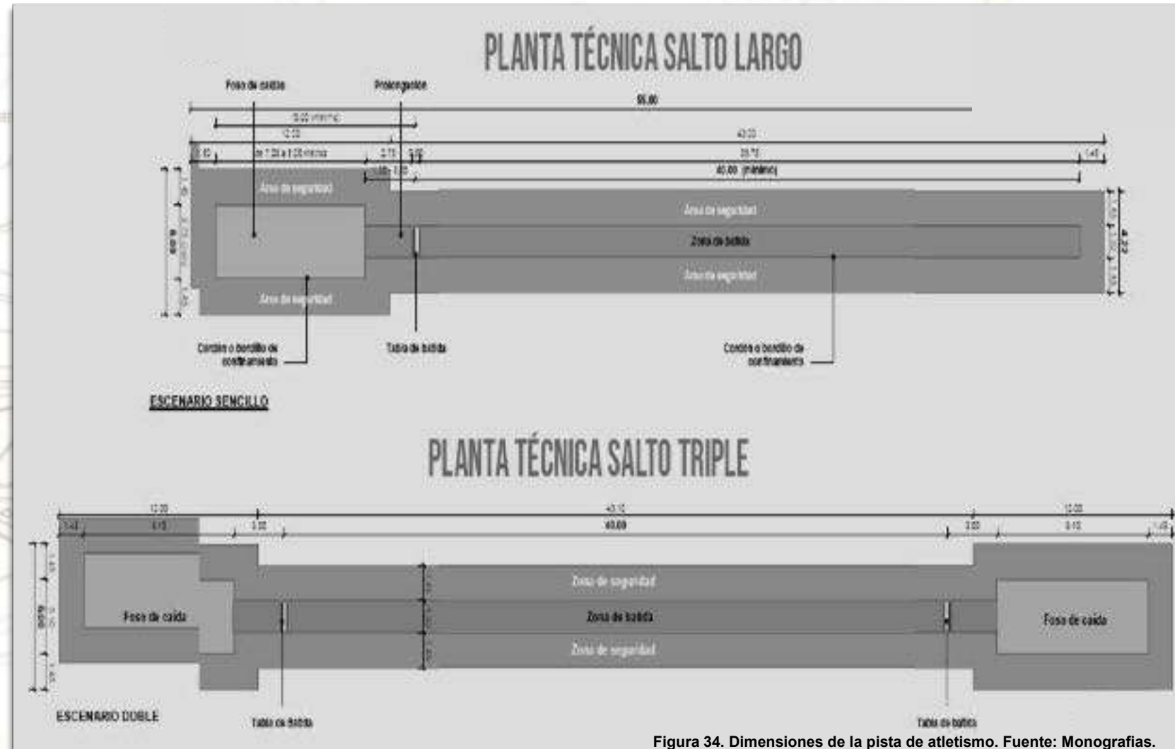
Figura 34. Dimensiones de la pista de atletismo. Fuente: Monografias.
