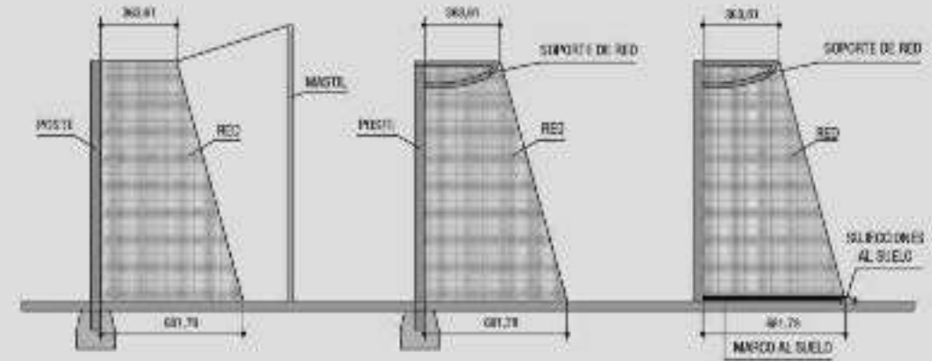
Figura 32. Postes y Red. Fuente: Manual instalaciones deportivas Navarra.
