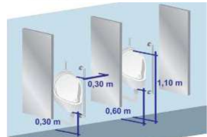
Figura 47. Orinales accesibles. Fuente: Coldeportes.
