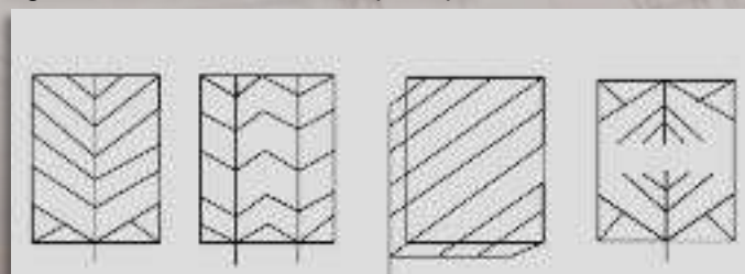
Figura 59. Tipo Espina de Pescado. Fuente: Estudio para el diseño de drenaje, riego y gramado de la cancha de fútbol del estadio.
