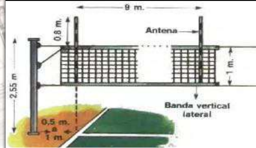
F7igura 7. Altura libre de obstáculos. Fuente: VoleibolenvenezuelaLA.
