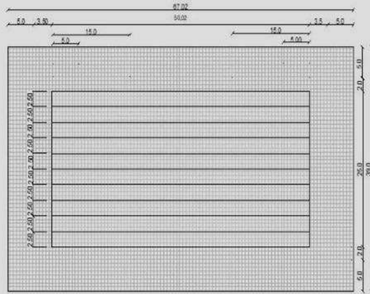
Figura 19. Dimensiones de competencia de carreras. Fuente: Oficina asesora de infraestructura – IDER.
