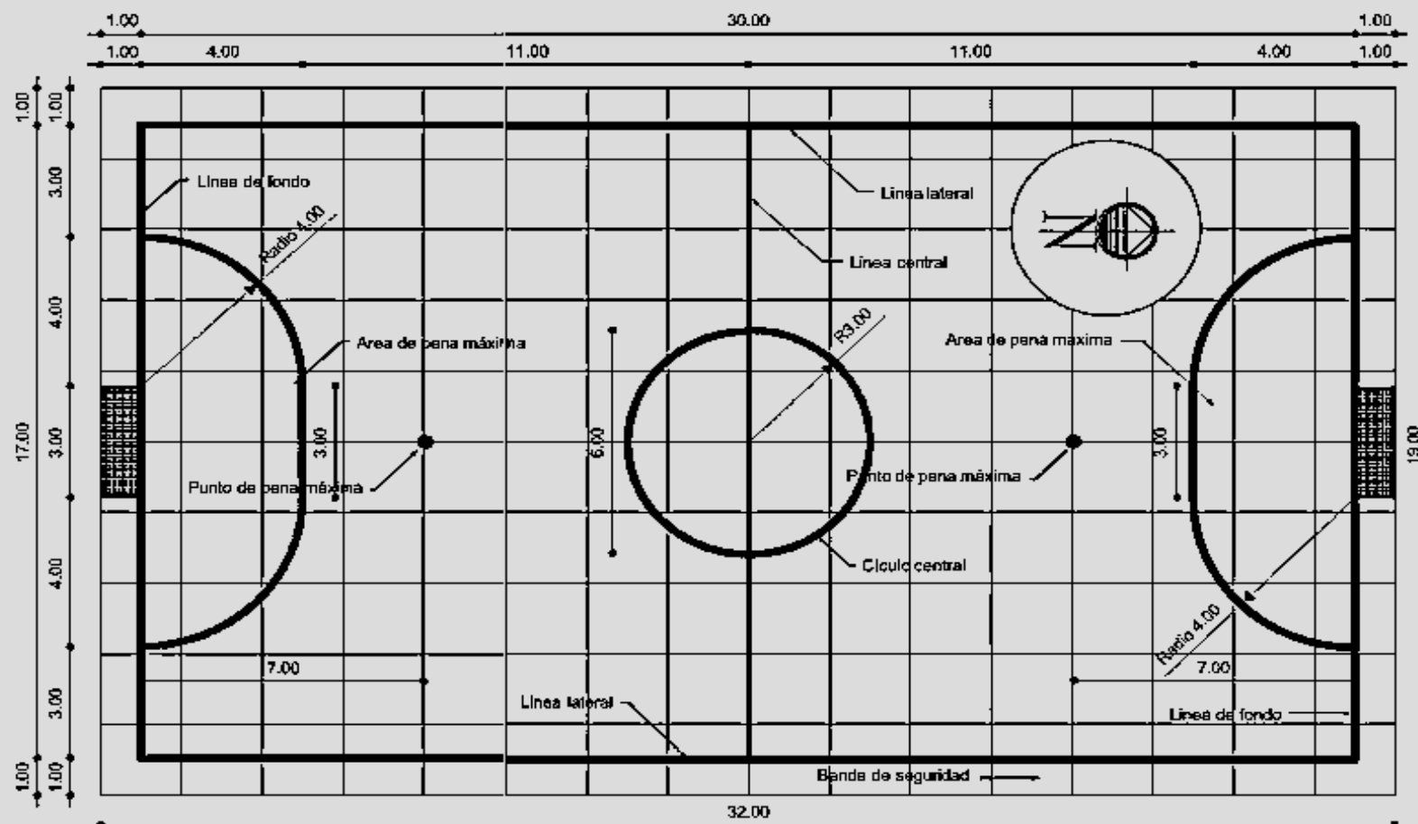
Figura 17. Dimensión Cancha microfútbol. Fuente: Parque y Grama.
