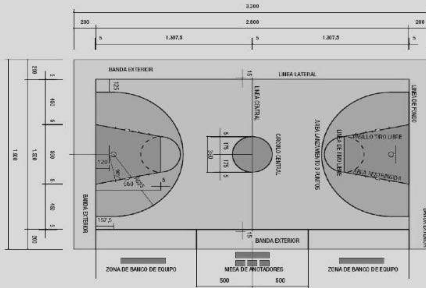
Figura 19. Medidas zona de juego baloncesto. Fuente: Manual instalaciones deportivas Navarra.
