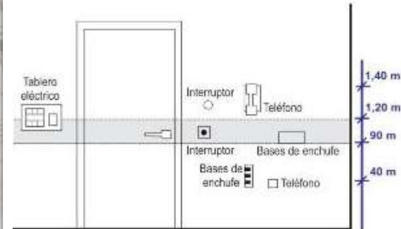
Figura 52. Interruptores y controles. Fuente: Coldeportes.
