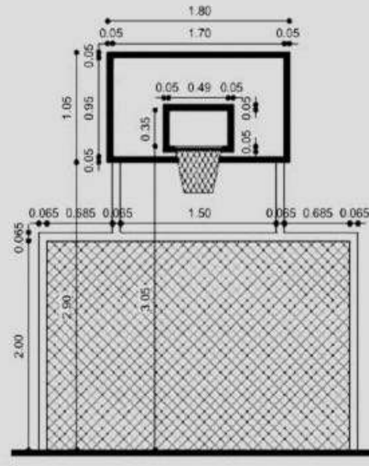
Figura 28. Vista frontal soporte integrado baloncesto y microfútbol. Fuente: Parque y Grama.
