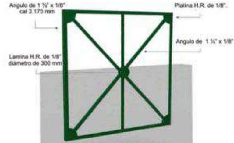
Figura 50. Estructura metálica panel. Fuente: Pag. Web IDRD.
