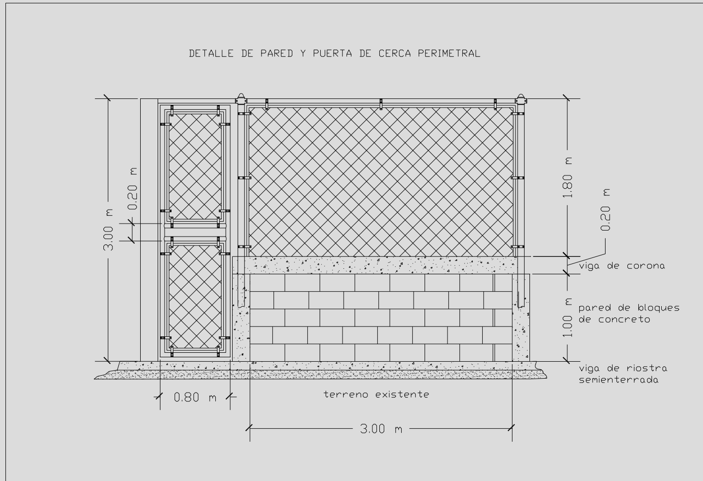
Figura 45. Cerramiento Detalle de pared. Fuente: Oficina asesora infraestructura – IDER.
