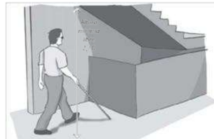
Figura 30. Espacios bajo escaleras, protegidas para evitar accidentes, altura mínima 2,10m. Fuente: Coldeportes.
