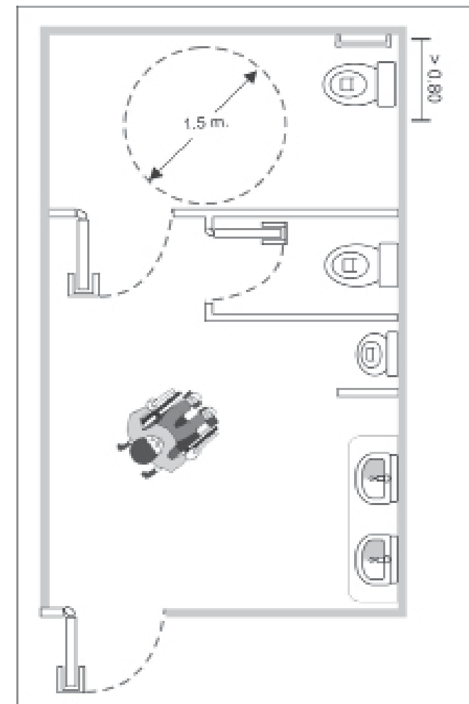
Figura 42. Batería Sanitaria. Fuente: Coldeportes.
