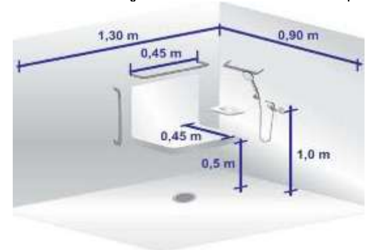
Figura 48. Duchas accesibles. Fuente: Coldeportes.
