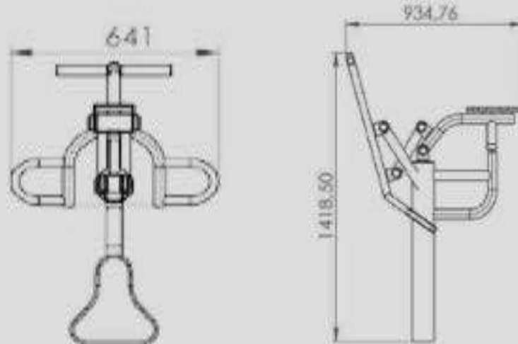
Figura 32. Dimensiones El Pony. Fuente: Equidesa.
