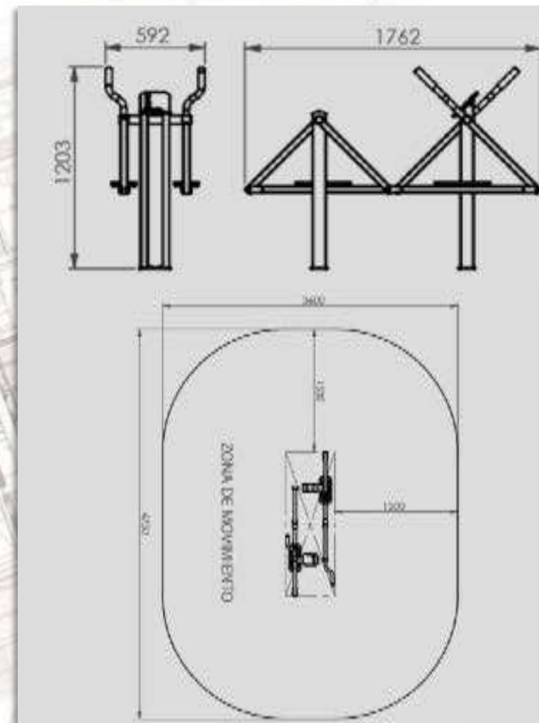
Figura 38. Dimensiones Esquí de Fondo ó Andador. Fuente: Equidesa.
