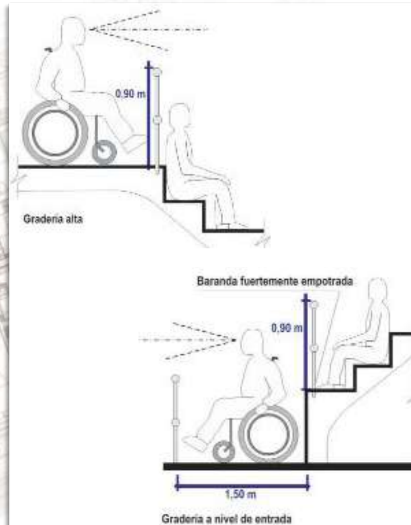
Figura 71. Graderías Accesibles. Fuente: Coldeportes.
