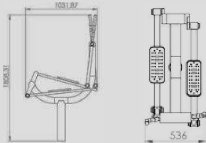
Figura 30. Dimensiones El Esquí. Fuente: Equidesa.
