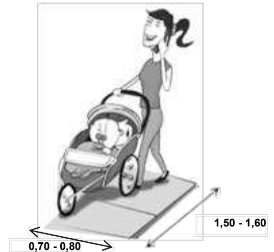
Figura 12. Persona con coche para bebé. Fuente: Coldeportes.
