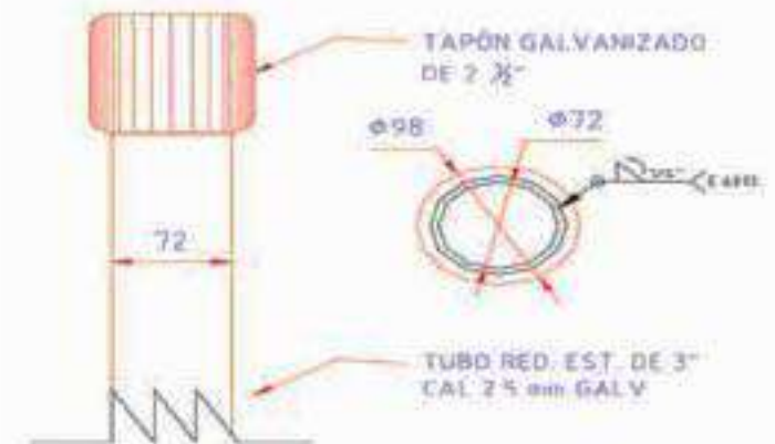
Figura 47 Detalle Soldadura Tapón. Fuente: Pag. Web IDRD.
