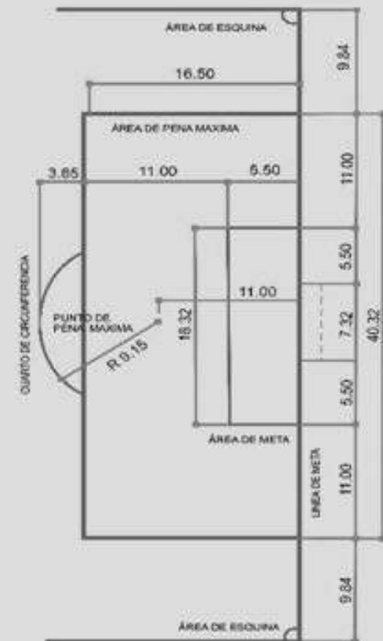
Figura 32. Áreas del Campo. Fuente: Manual instalaciones deportivas Navarra.
