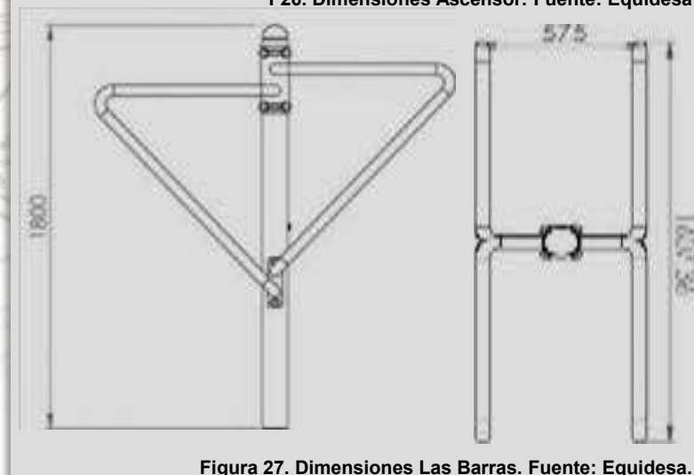
Figura 27. Dimensiones Las Barras. Fuente: Equidesa.
