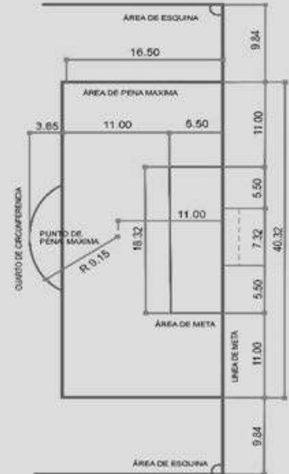
Figura 18. Áreas del Campo. Fuente: Manual instalaciones deportivas Navarra.
