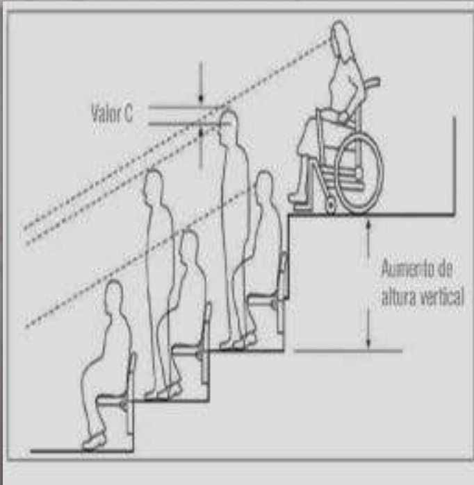
Figura 1. Línea de Visión. Fuente: Instituto de biomédica Valencia.
