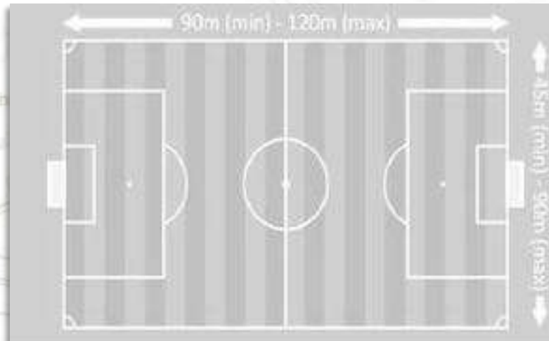
Figura 19. Futbol 11. Fuente: Pinterest.
