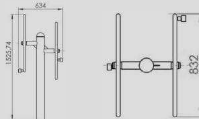
Figura 35. Dimensiones El Timón. Fuente: Equidesa.
