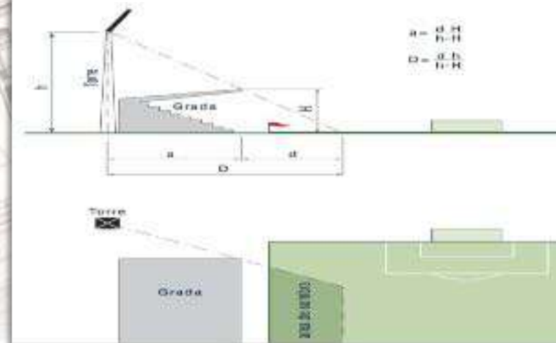
Figura 11. Altura de torres limitadas por graderías. Fuente: Indal.
