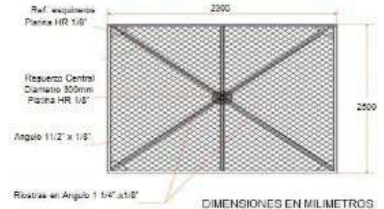
Figura 52. Panel . Fuente: Pag. Web IDRD.
