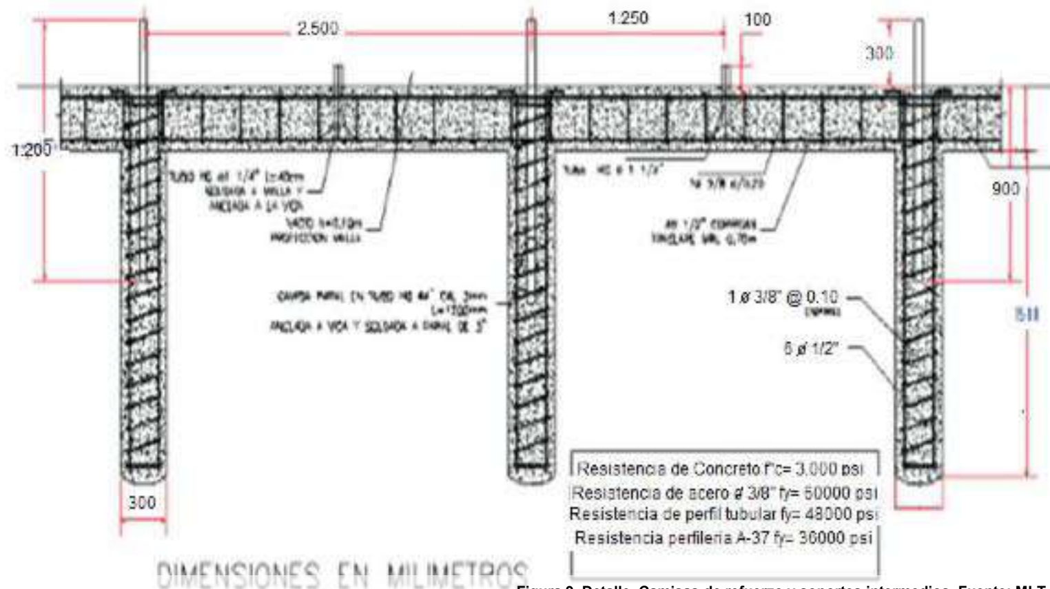
Figura 9. Detalle Camisas de refuerzo y soportes intermedios. Fuente: MLT IDRD.
