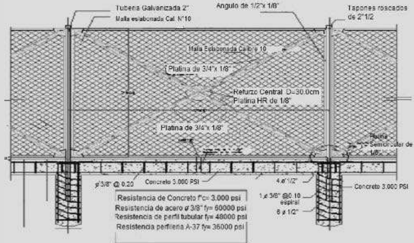
Figura 48. Cerramiento Malla eslabonada y concreto reforzado. Fuente : Pag. Web IDR.
