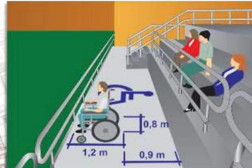
Figura 69. Dimensiones graderías accesibles. Fuente: Coldeportes.
