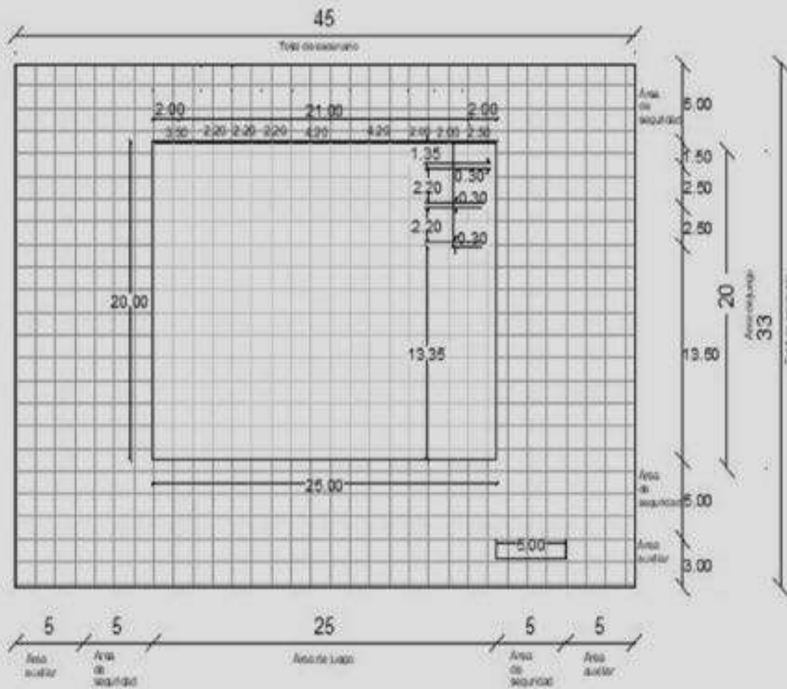
Figura 18. Dimensiones de competencia de salto. Fuente: Oficina asesora de infraestructura – IDER.
