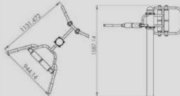
Figura 33. Dimensiones El Masaje. Fuente: Equidesa.
