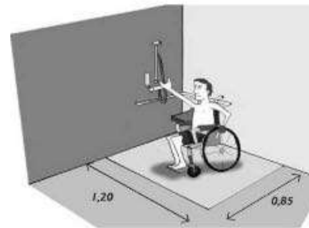
Figura 44. Duchas. Fuente: Coldeportes.
