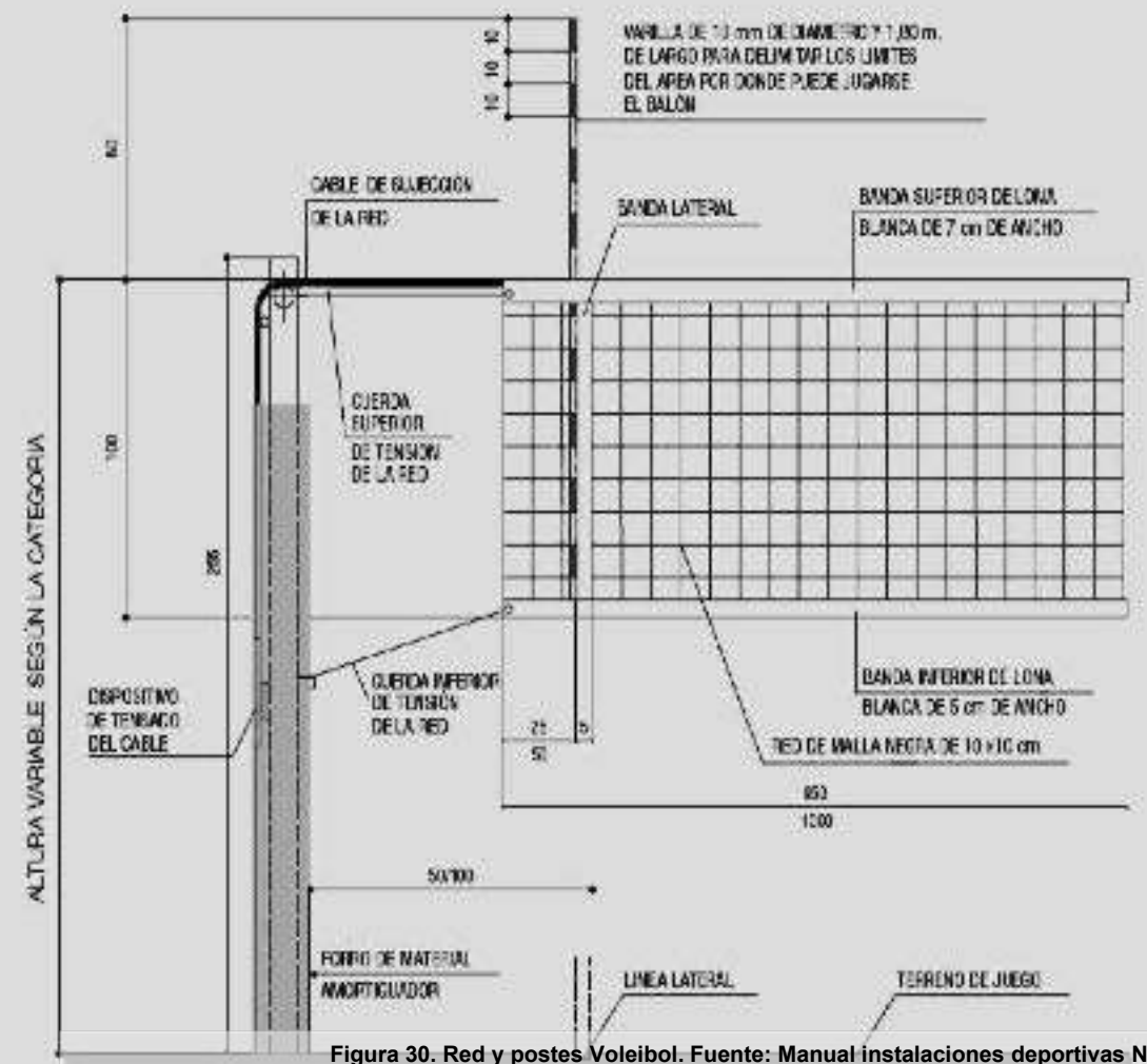
Figura 30. Red y postes Voleibol. Fuente: Manual instalaciones deportivas Navarra.
