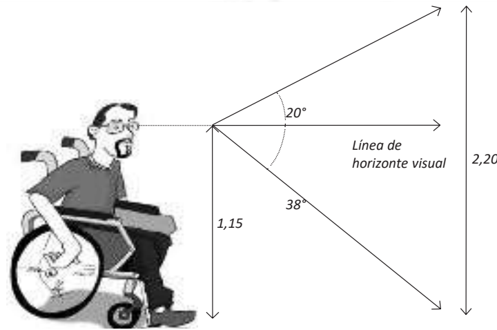
Figura 17. Visual de una persona en silla de ruedas. Fuente: Coldeportes.
