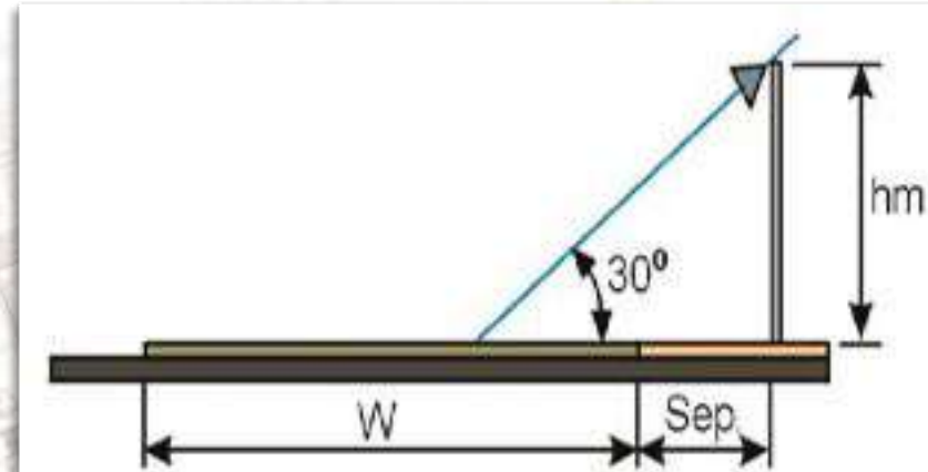
Figura 10. Relación entre la separación del campo y la altura de los postes. Fuente: Retilap 560.3.3.
