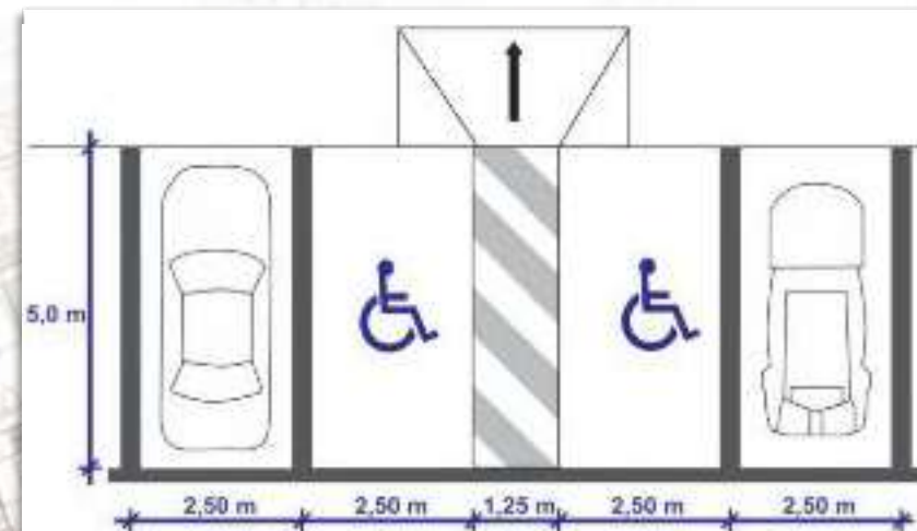
Figura 35. Estacionamientos. Fuente: Coldeportes.
