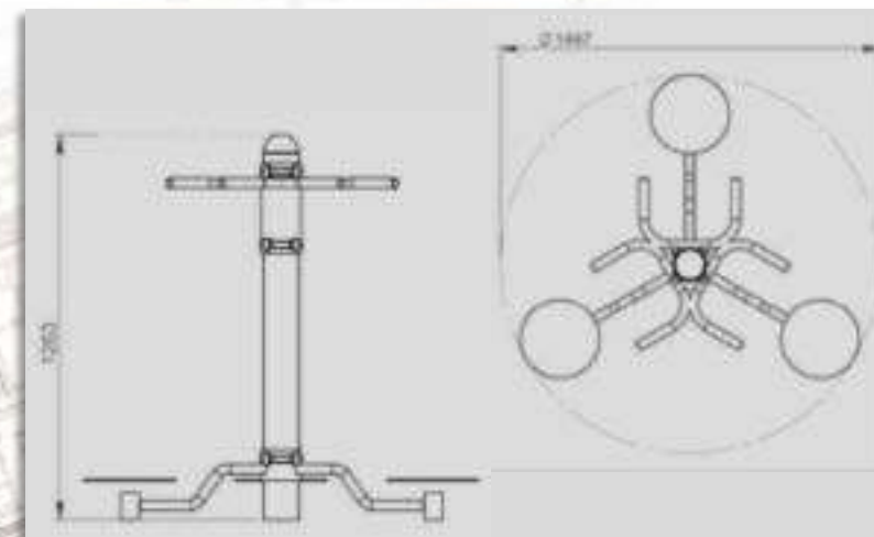
Figura 28. Dimensiones La Cintura. Fuente: Equidesa.
