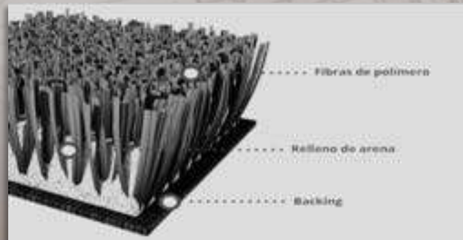
Figura 7. Partes de un césped artificial. Fuente: Siaver.
