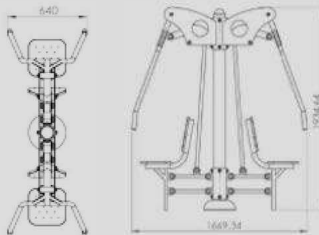
Figura 37. Dimensiones El Caballo. Fuente: Equidesa.
