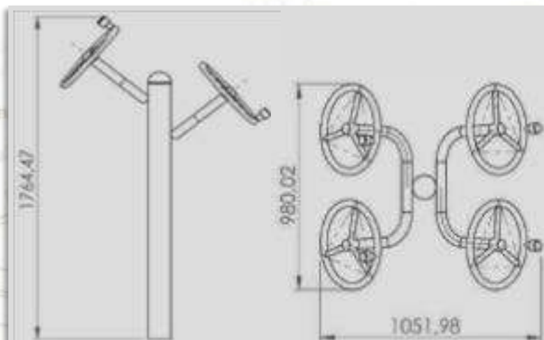
Figura 36. Dimensiones El Volante. Fuente: Equidesa.
