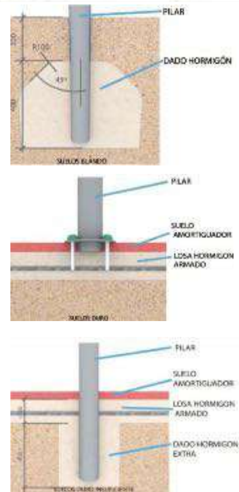
Figura 25. Ficha Técnica Instalación Maquinas Biopsaludables. Fuente: Equidesa.
