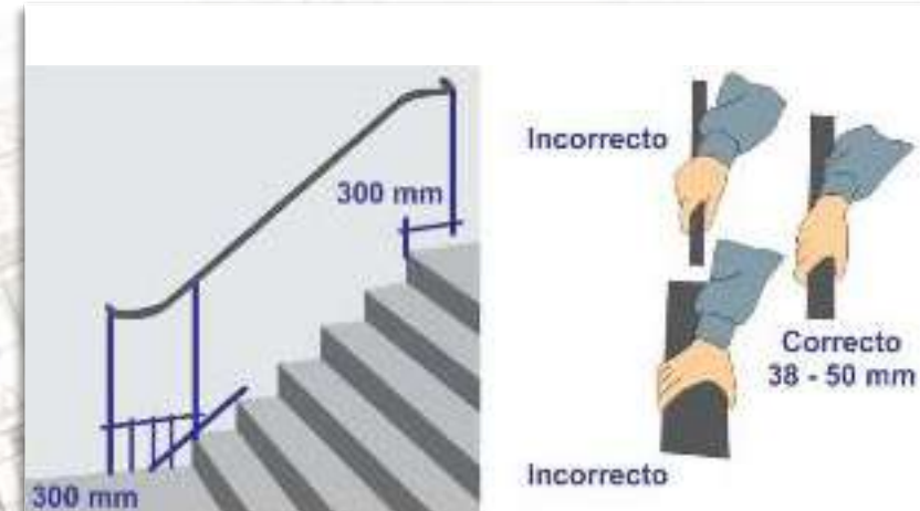
Figura 31. Pasamanos. Fuente: Coldeportes.
