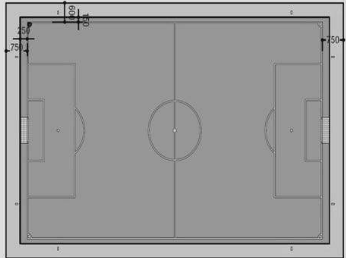
Figura 16. 1Ra División e Internacionales. Fuente: Manual instalaciones deportivas Navarra.
