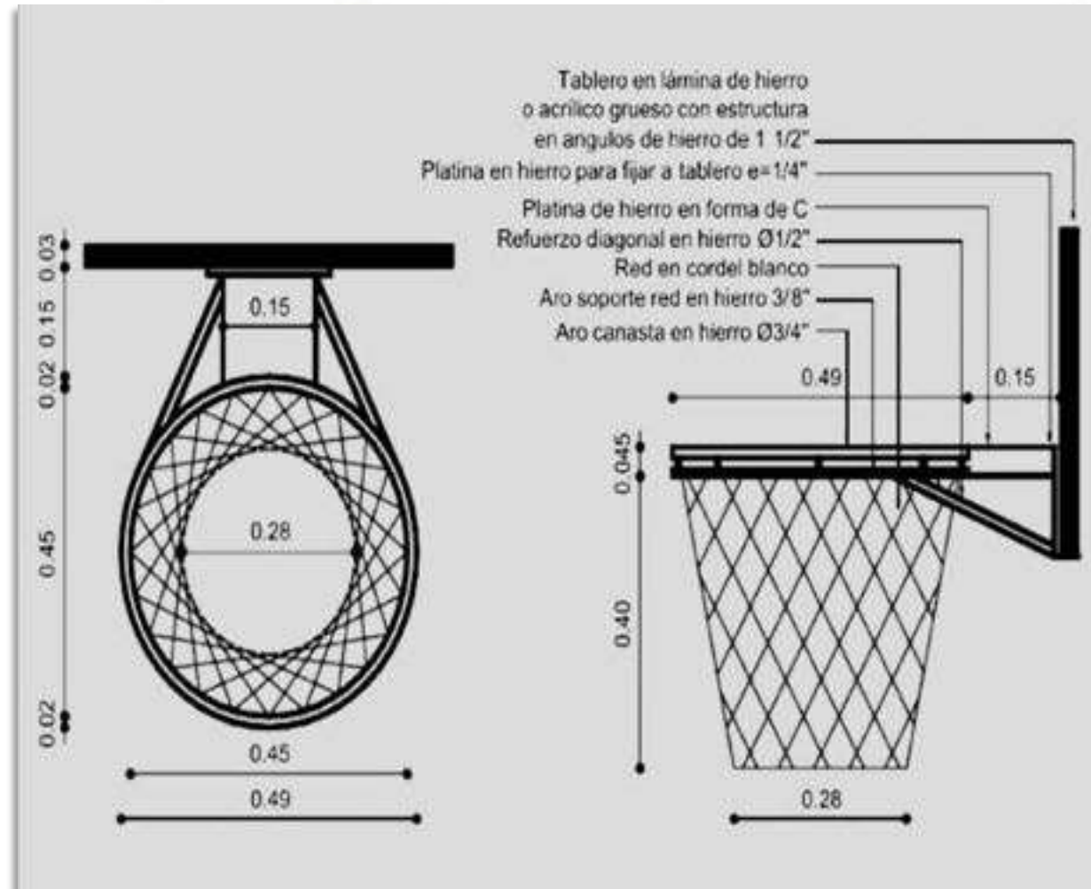
Figura 29. Tablero y aro Baloncesto. Fuente: Parque y Grama.
